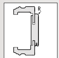
PZ-4 R Ausführung profilierte Beklei- dungen, runde Futterplatte
