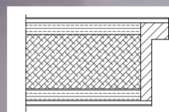
gefälzte Kante mit Einleimer aus Massivholz
