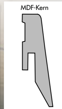
MDF-Kern MEISTER Profil 3 PK 20 x 60 mm
